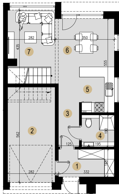
RZUT PARTERU
