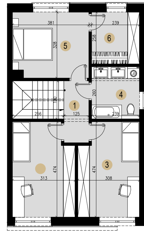
RZUT PIĘTRA
