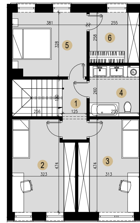
RZUT PIĘTRA
